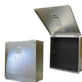
Meter Box CLSOL GALV 450x450x270mm
